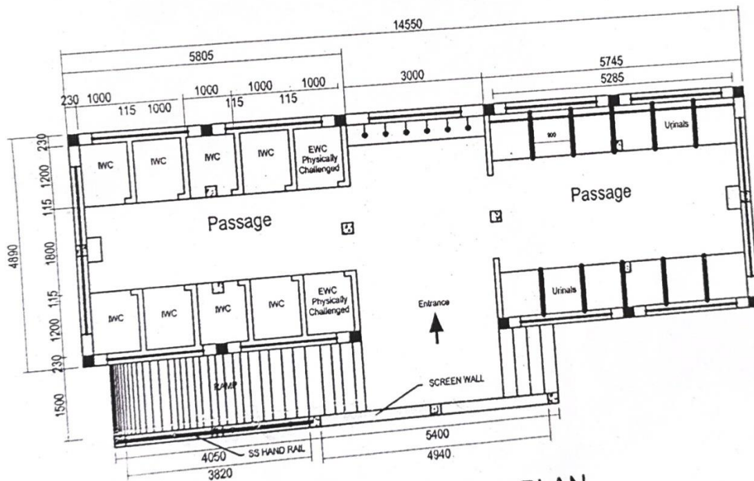
LADIES TOILET - PLAN
